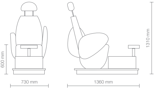
DIMENSIONI (mm) - DIMENSIONS (mm)
